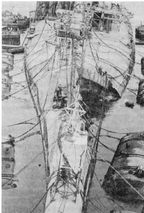
Рис. 3. Вид на пробоину в днище линкора «Новороссийск»
