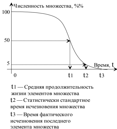
Рис. 7. ХАРАКТЕР УБЫЛИ ЭЛЕМЕНТОВ ИЗ ПЕРВОНАЧАЛЬНОГО СОСТАВА МНОЖЕСТВА С ТЕЧЕНИЕМ ВРЕМЕНИ
