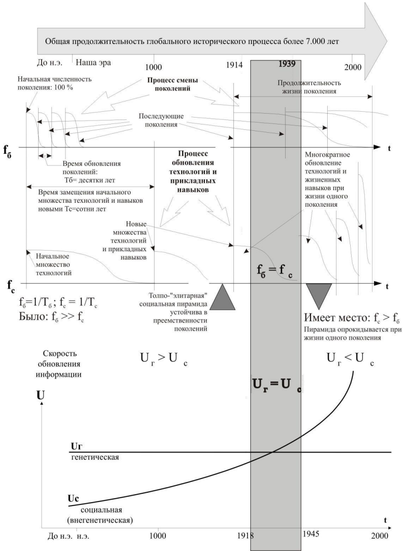
Рис. 8. Изменение соотношения эталонных частот биологического и социального времени
