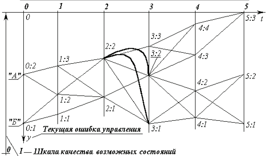
Рис. 7. ДИНАМИЧЕСКОЕ ПРОГРАММИРОВАНИЕ,
