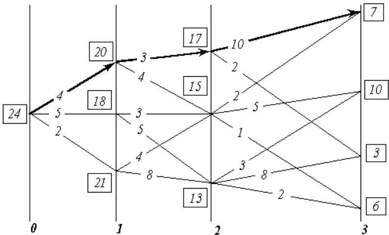
Рис. 10. К СУЩЕСТВУ МЕТОДА ДИНАМИЧЕСКОГО ПРОГРАММИРОВАНИЯ. ОПТИМАЛЬНАЯ ТРАЕКТОРИЯ.
