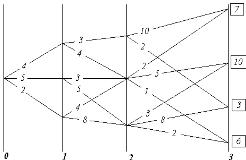
Рис. 8. К СУЩЕСТВУ МЕТОДА ДИНАМИЧЕСКОГО ПРОГРАММИРОВАНИЯ. МАТРИЦА ВОЗМОЖНОСТЕЙ.
