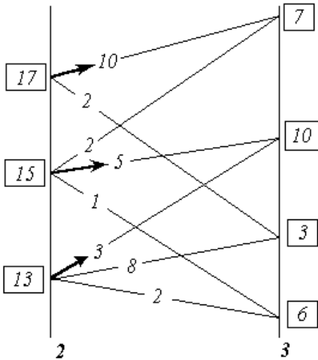
Рис. 9. К СУЩЕСТВУ МЕТОДА ДИНАМИЧЕСКОГО ПРОГРАММИРОВАНИЯ. АНАЛИЗ ПЕРЕХОДОВ.
